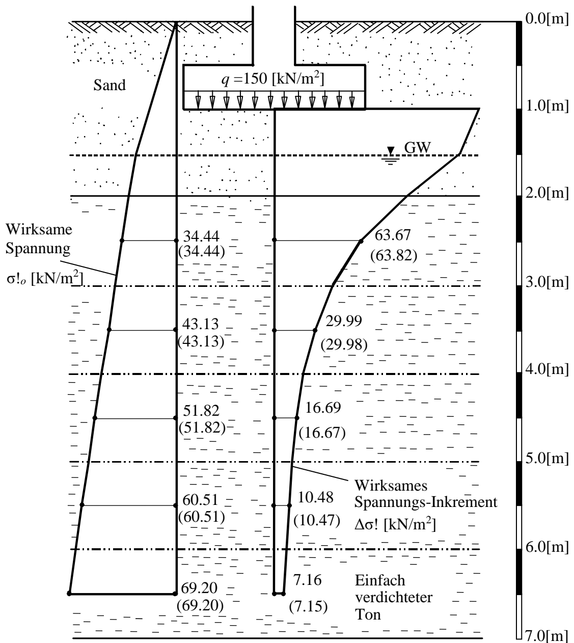
Bild 9 Wirksame Spannung \sigma'_o [kN/m²] und wirksames Spannungskrement \Delta\sigma' [kN/m²] (Ergebnisse \Delta\sigma' gerechnet mit ELPLA , Handberechnung in Klammern)
